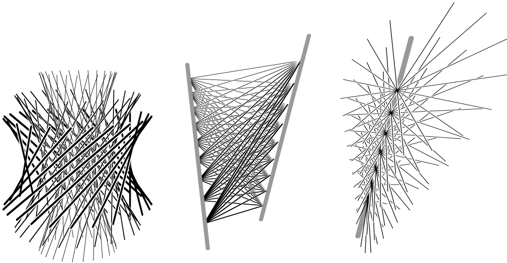
Abbildung 1: Von links nach rechts: elliptisches, hyperbolisches und parabolisches Netz.
