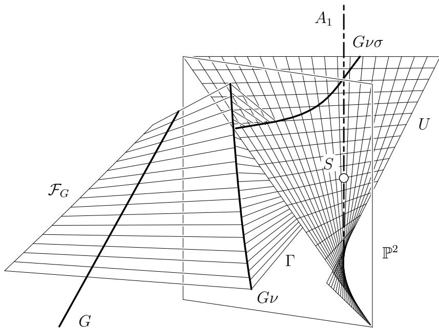
Abbildung 3: Zerlegung der hyperbolischen linearen Geradenabbildung.
