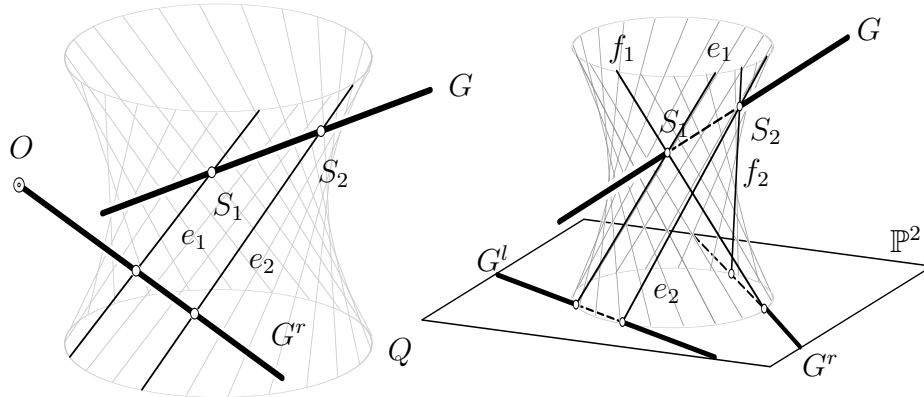
Abbildung 7: Geradenabbildung nach ECKHART (links) und nach REHBOCK (rechts).
