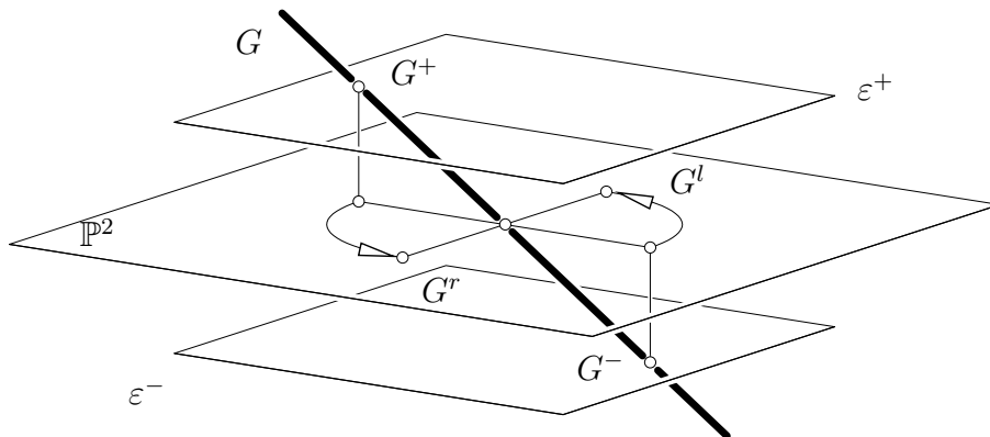
Abbildung 5: Kinematische Abbildung von BLASCHKE und GRÜNWARD.
