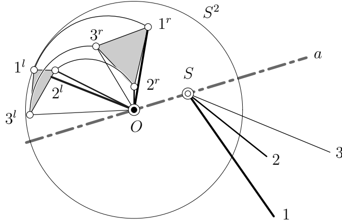
Abbildung 6: Sphärisch kinematisches Bild eines Dreikants.
