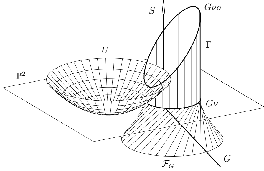
Abbildung 2: Zerlegung der elliptischen linearen Geradenabbildung.
